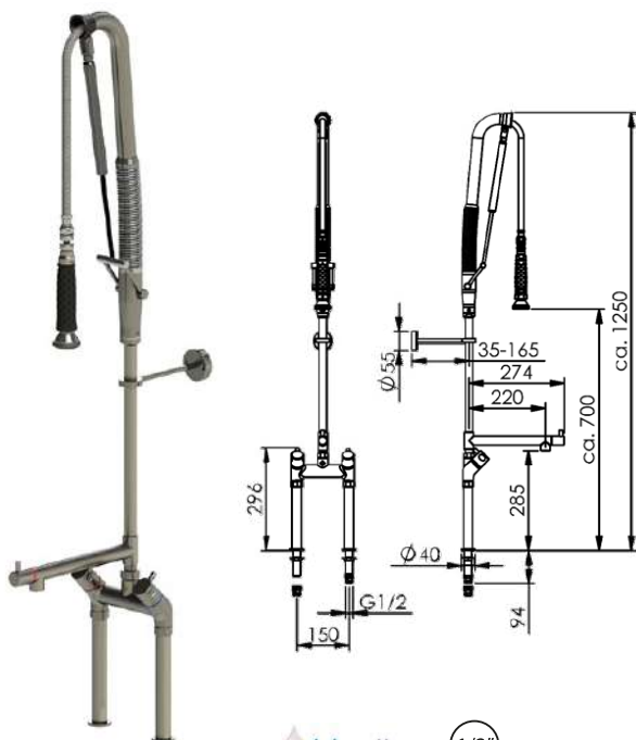
Bateria prysznicowa; Stal nierdzewna 316 L Pre-rinse unit; 316 L Stainless steel
