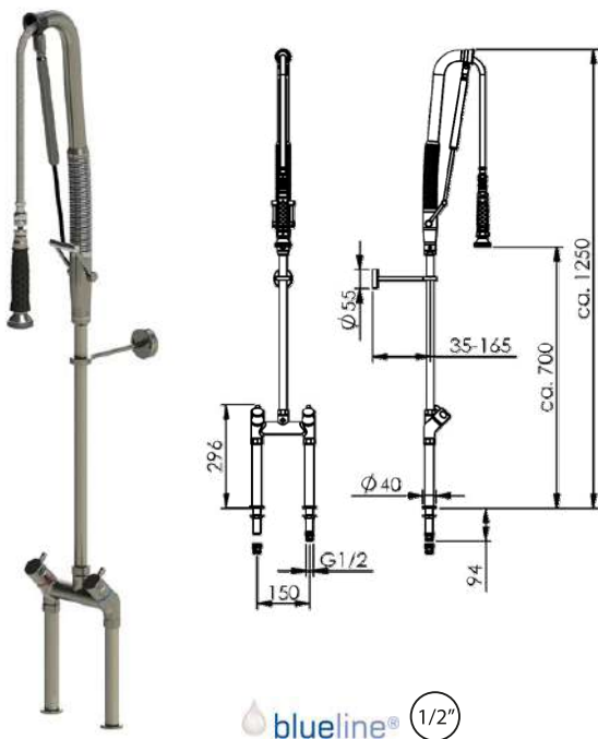
Bateria prysznicowa; Stal nierdzewna 316 L Pre-rinse unit; 316 L Stainless steel
